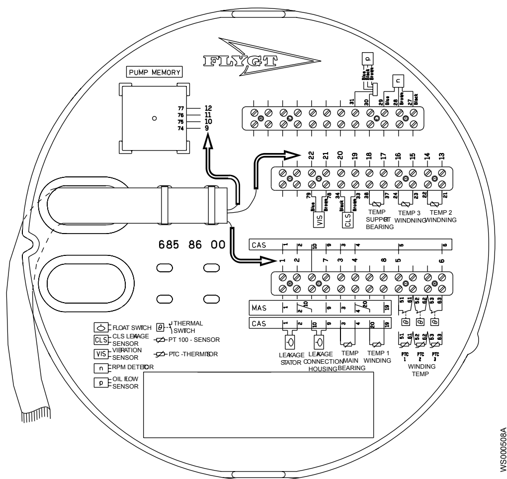
Рис. 22: MAS 711, стрелки указывают номера проводов кабеля SUBCAB
