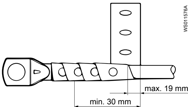
Рис. 14: Использование изоляционной ленты
