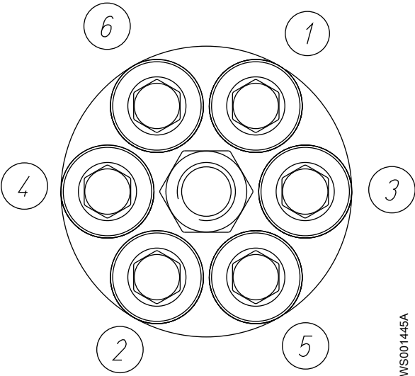
Рис. 34: Диагональный рисунок для периферийных винтов
