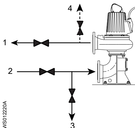
Рис. 9: Перекройте вентиляционные клапаны в кожухе (показаны типовые насосы)
